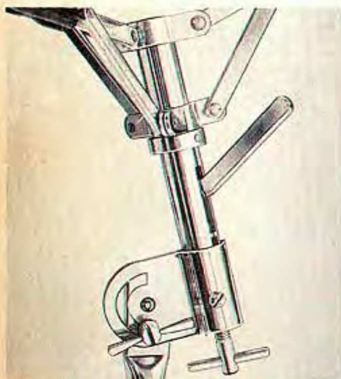
Z 5553 Trommelständer „Champion“ Die Tragarme brauchen nur einmal auf den Trommel- durchmesser eingestellt werden und können dann stets durch einfachen Hebeldruck festgestellt oder gelöst werden (DGM)
