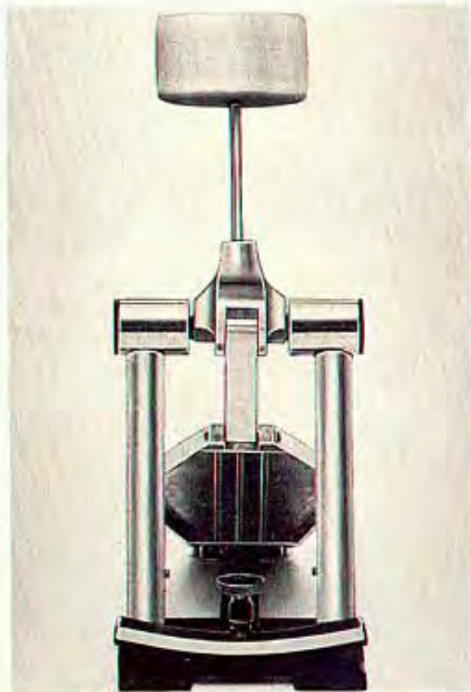
Z 5319 Fußmaschine „Champion“ Exzentrischer Bewegungsablauf, regulierbare Zugfedern in Säulen eingelassen, doppelte Kugellagerung, Metallzugband, breiter Klemmbügel
