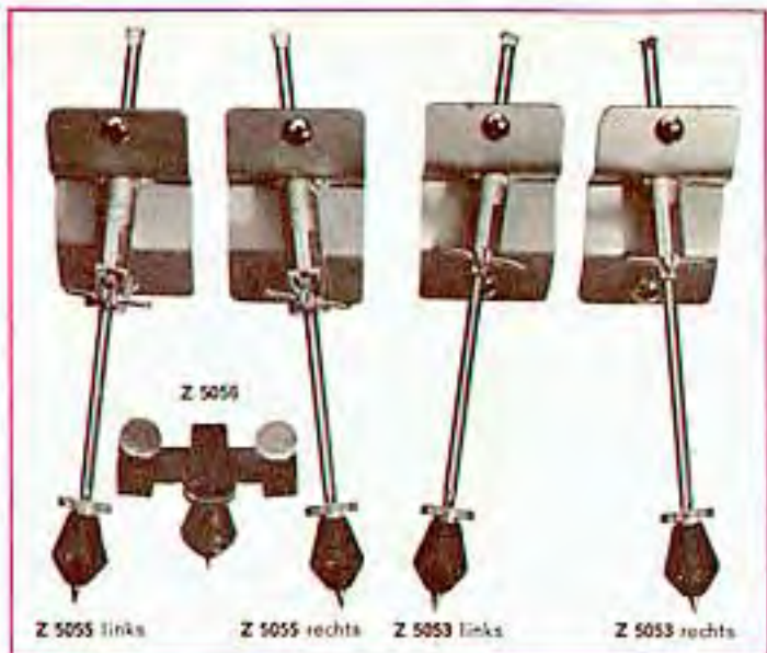
Feststellspitzen, auf Gummi- oder Metallspitze umstellbar Z 5053 mit Druckschraube Z 5055 mit Klemmschraube Z 5056 Feststellhorn für Große Trommel
