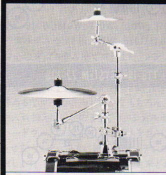
CH712+CSAT910 ●クローズハイハット CH712+CSAT914 ●1シンバル
