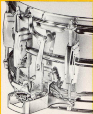
P-88 STRAINER
