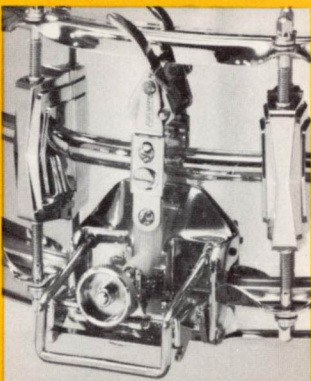
P-70 STRAINER
